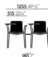
HAL Tube Writing Tablet con elemento di raccordo per file di sedie
