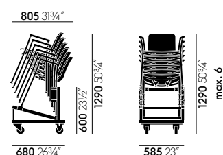
HAL RE Tube Armrest, base in tubolare d'acciaio a quattro gambe, impilabile
