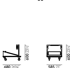
HAL Carrello di impilaggio, adatto a tutti i modelli di sedie HAL impilabili
